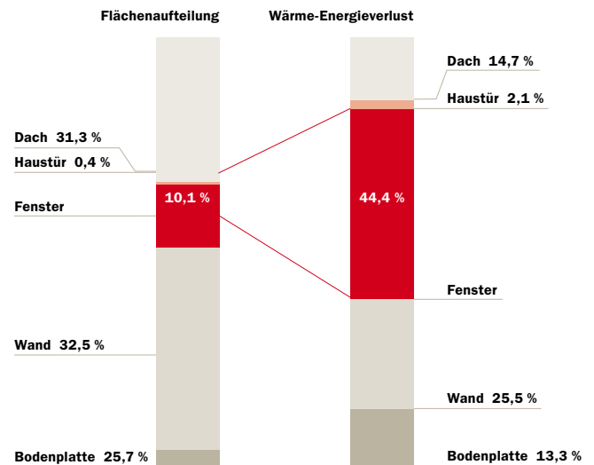
Wärme-Energieverluste am Beispiel eines Einfamilienhauses mit einer Fläche von 525 m 2 Gebäudehülle
